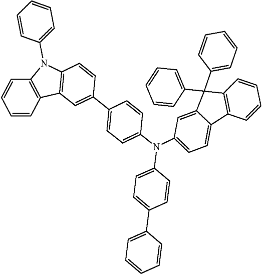
HT5
