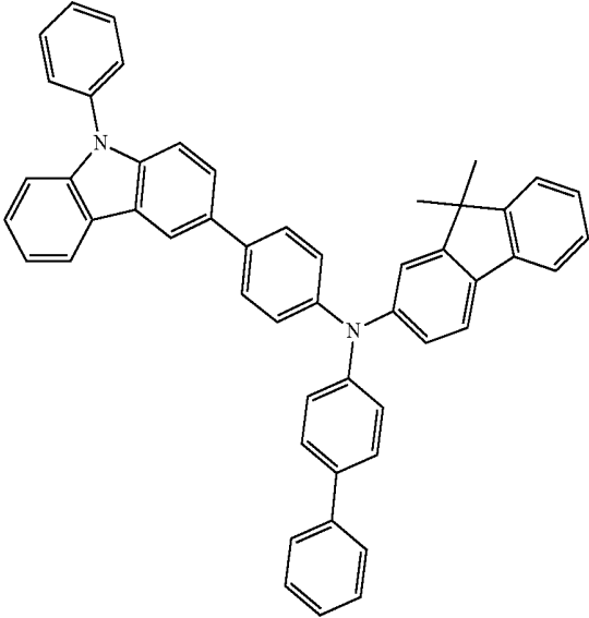
HT3
