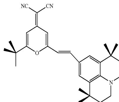
DCJTb
