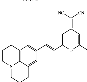
DCM
