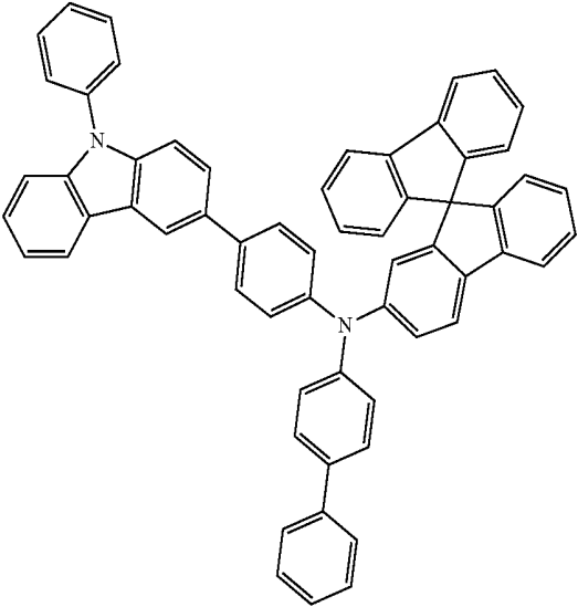
HT6
