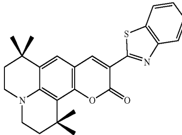
C545T
